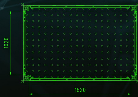
A-A (Arbeitsraum)
